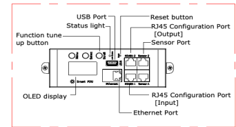
DETAIL A 1.5:1
